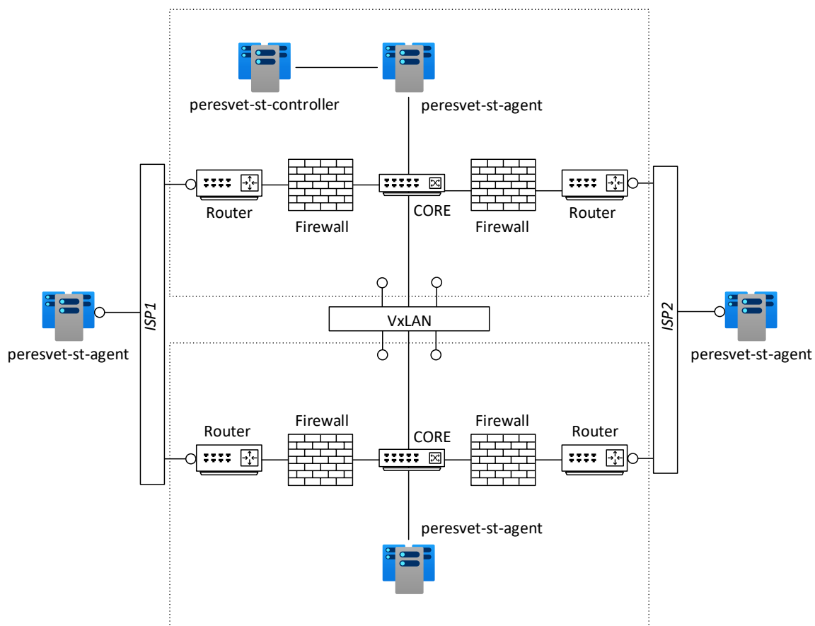
Рис. 12 – Схема использования Пересвет-СТ
